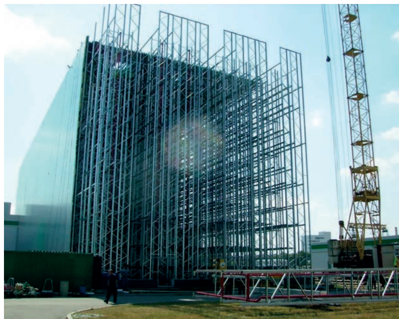
Монтаж м/к корпусу та обладнання роботизованого складу фармацевтичної компанії «Дарниця» (Україна, м.Київ)
